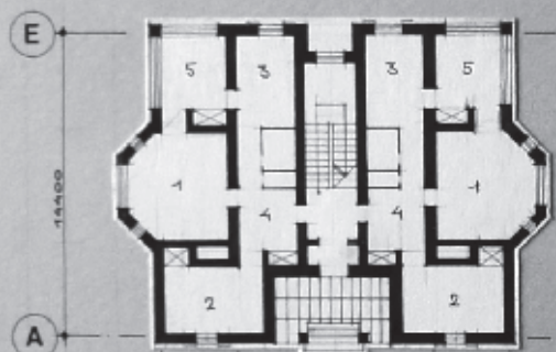
ПЛАН 1 ЭТАЖА
