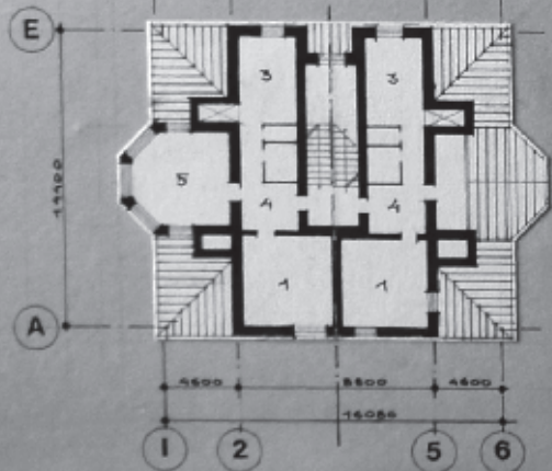
ПЛАН 2 ЭТАЖА
